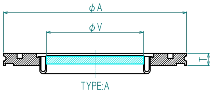
ISOフランジ用ビューポート【溶接タイプ】
