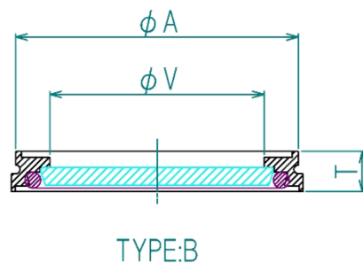
ISOフランジ用ビューポート【Oリングタイプ】
